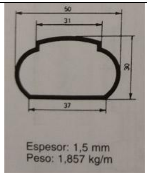
PASAMANOS DECORATIVO 1
