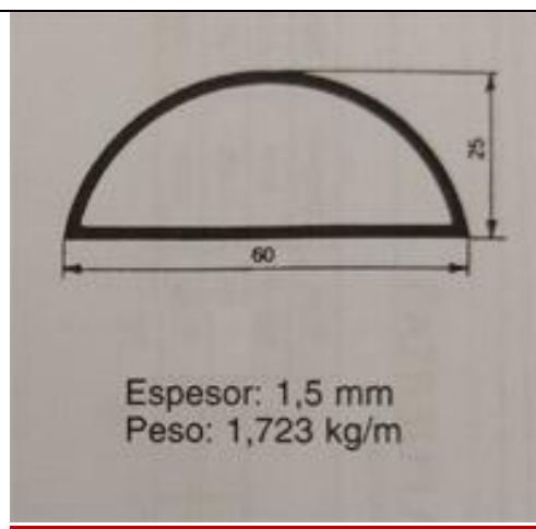
PASAMANOS DE 60
